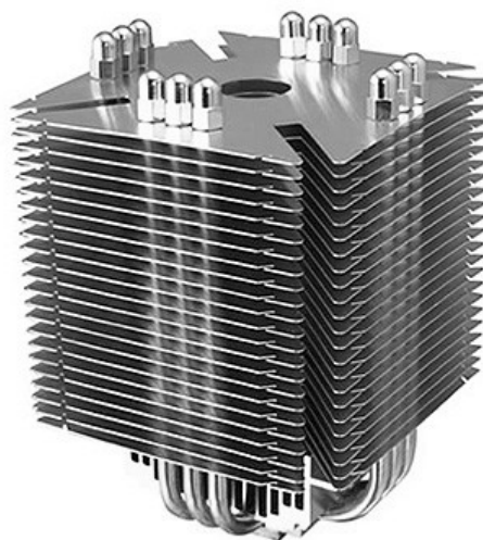
Obrázek 3: Chladič Scythe Ninja Masivní žebrování v kombinaci s technologií heatpipe dokáže pasivně uchladiť mnoho procesorů. Nevýhodami tohoto chladiče jsou ale velké rozměry a hmotnost přesahující oficiální nosnost základních desek.
